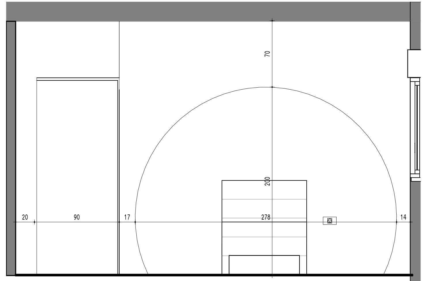
N-1 1 : 25
