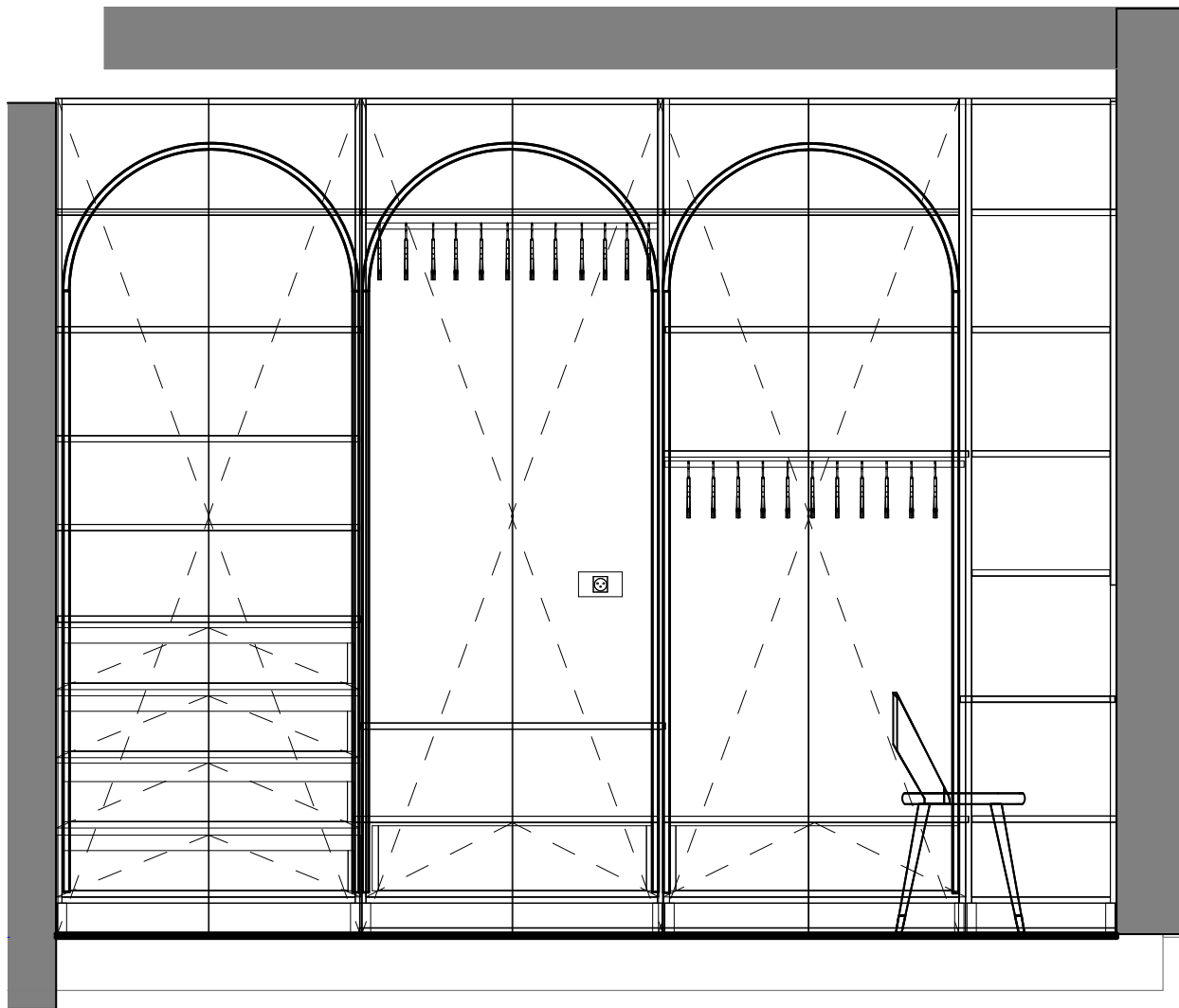
N2 1 : 25
