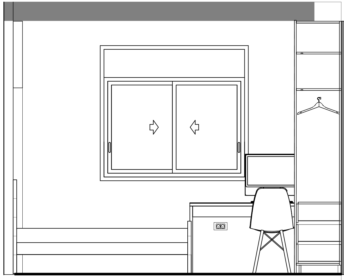
N-2 1 : 25
