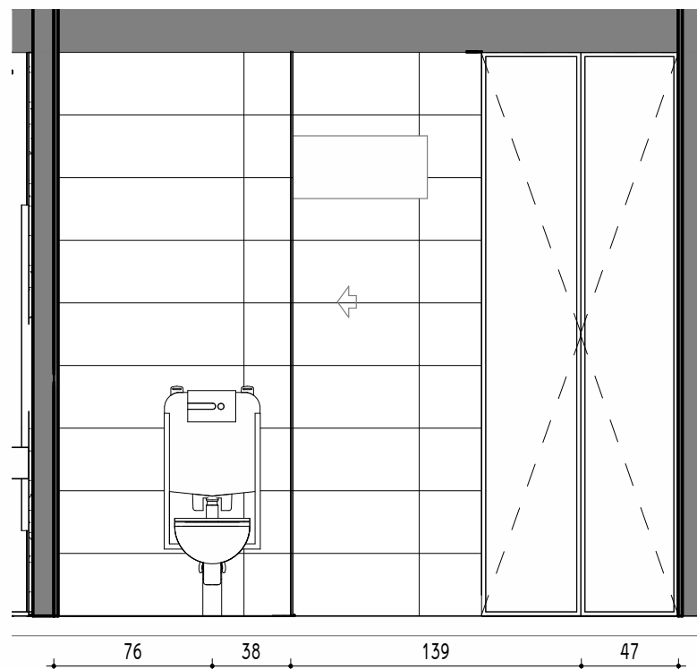
B2 1 : 35
