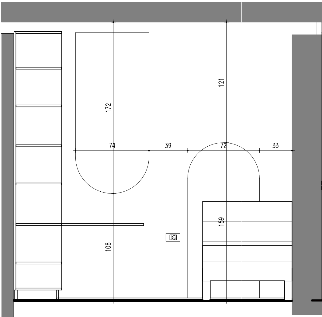
N1 1 : 25
