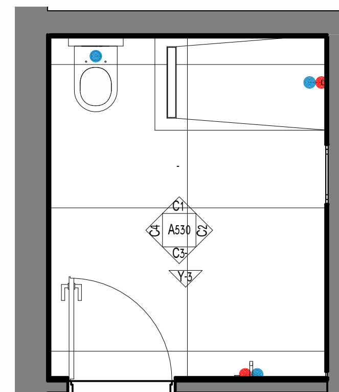
00 אינסטלציה 3 Callout - 1 : 35
