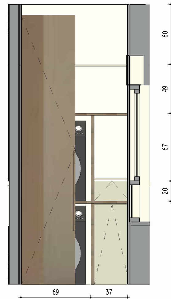
Y-7 1 : 25
