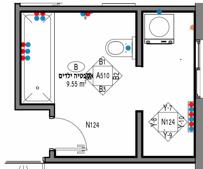
00 אינסטלציה 1 - Callout 1 : 50
