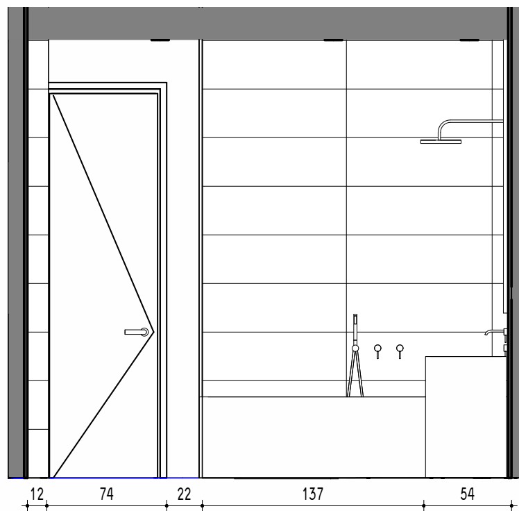
B4 1 : 35
