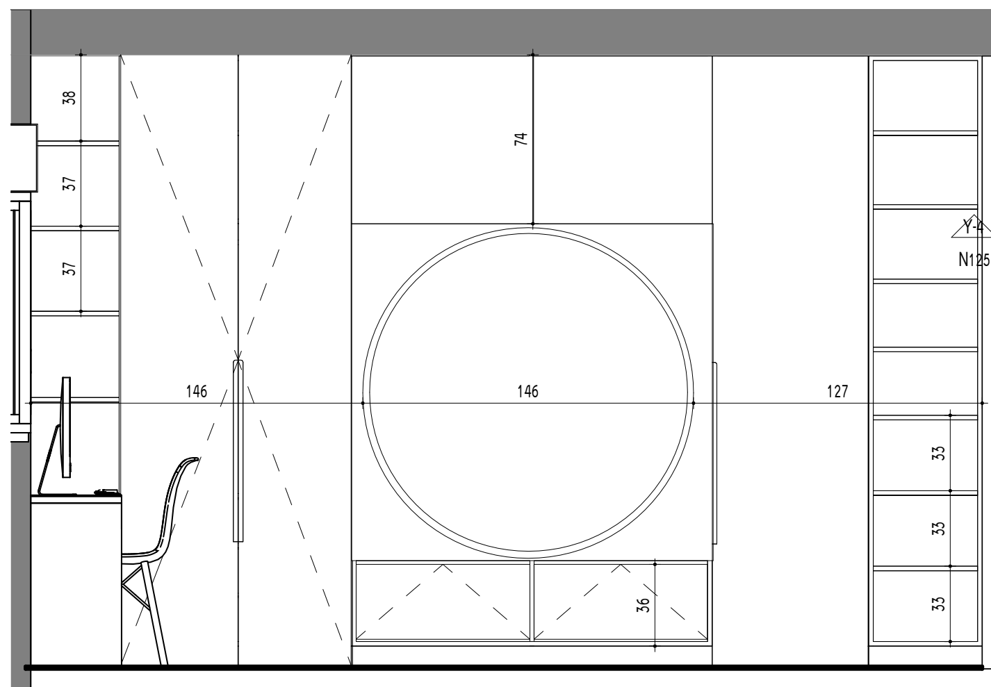
N-3 1 : 25
