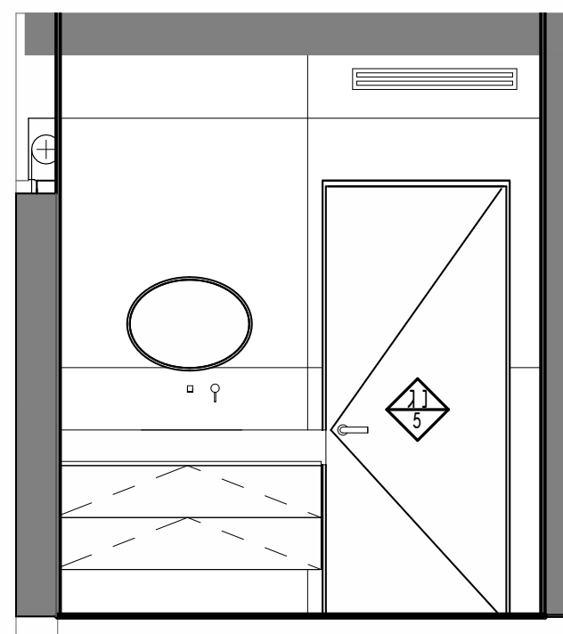
C3 1 : 35
