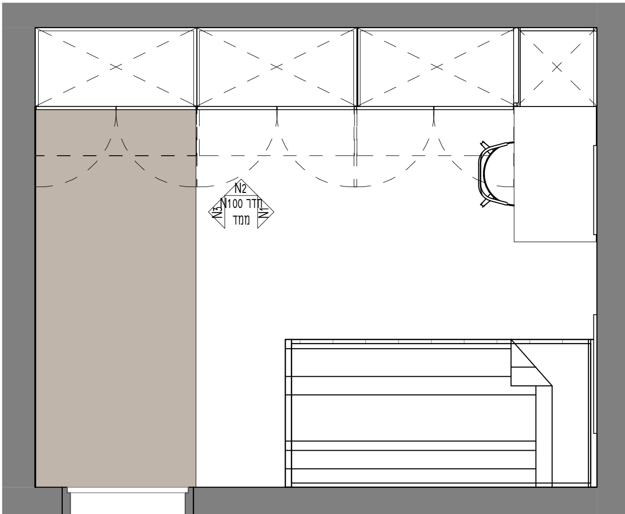
חדר ממד 1 : 25
